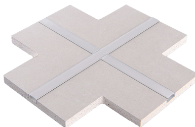
401067 Connettore a X Supporto in gesso Profilo alluminio Diff. smerigl.
